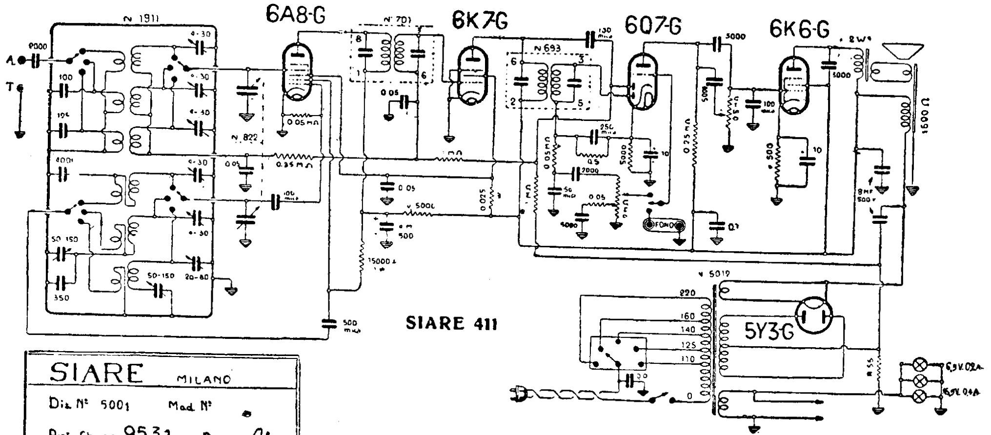
RADIO SIARE. — Mod. « 411 » prima serie. — Produzione 1938-39. — Gamme: cc. (17-30), c. (30-50), m. (210-520), l. (750-1800). — Media frequenza: 467 kHz.
